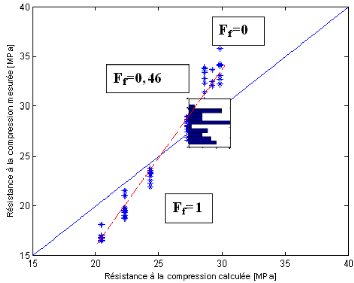
Figure 11. Comparaison entre valeurs calculées et mesurées de la résistance à la compression de bétons pour un dosage en ciment de 300 kg/m 3 et différents rapports eau/ciment.
