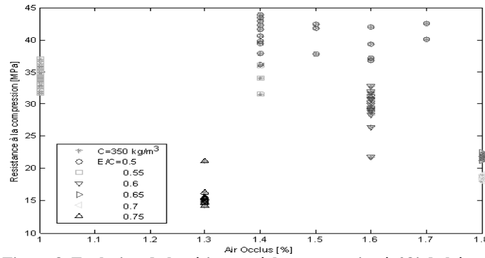
Figure 8. Evolution de la résistance à la compression à 28j de bétons conservés à l'eau pour un dosage en ciment de 350 kg/m 3 et différents rapports eau/ciment en fonction du pourcentage d'air occlus.
